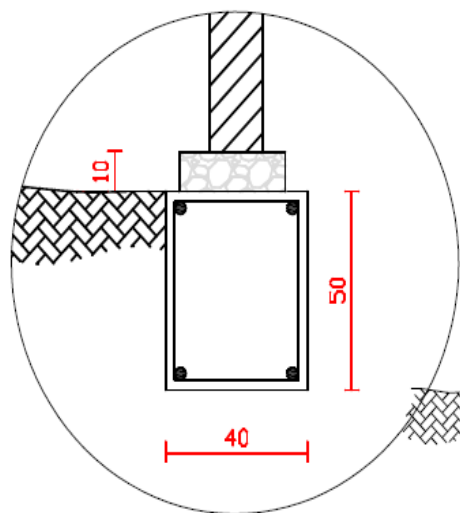
détails semelle
