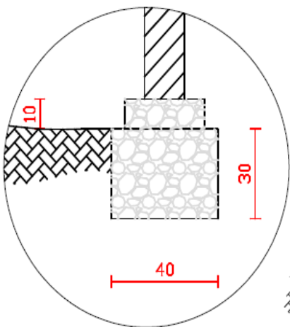
détails semelle
